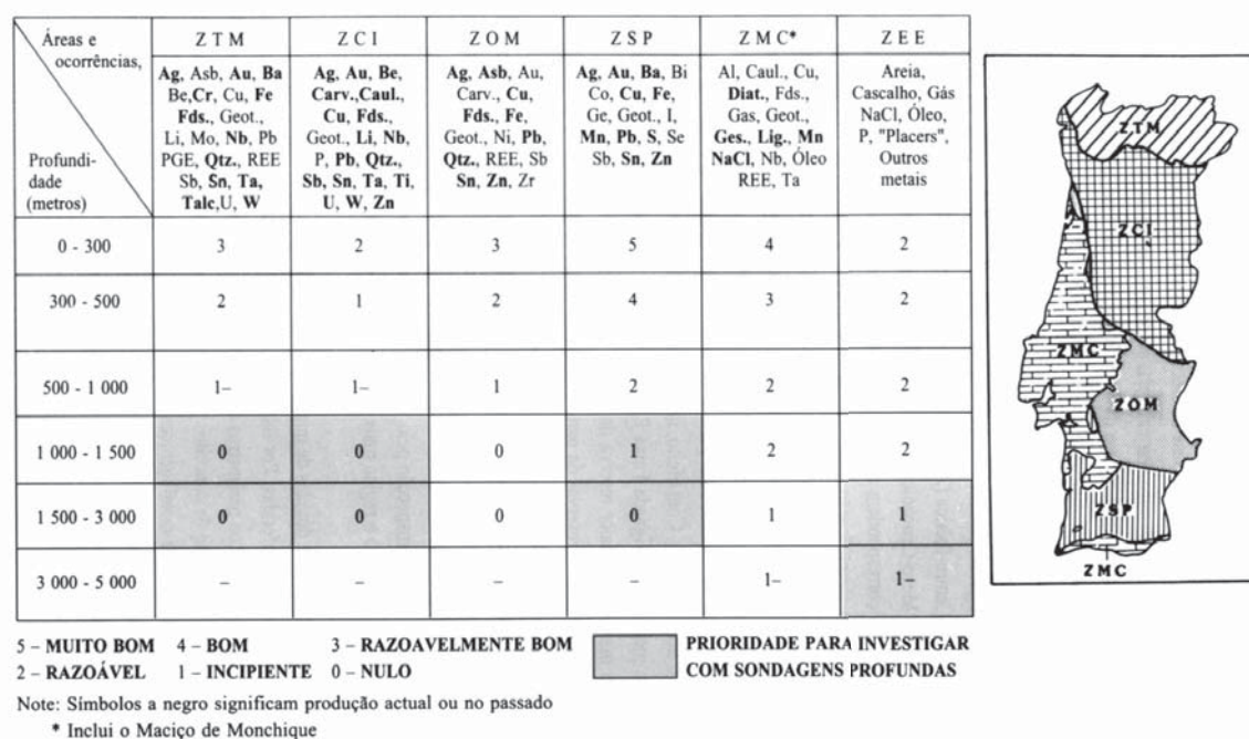
Figura 6 – Conhecimento Geocientífico da Base de Recursos para diferentes profundidades.
