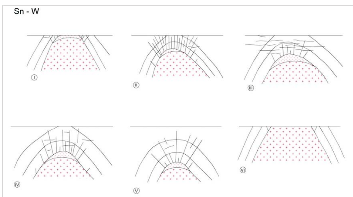
Figura 8 – Representação esquemática de granitos a diferentes profundidades e tipos de filões associados.
